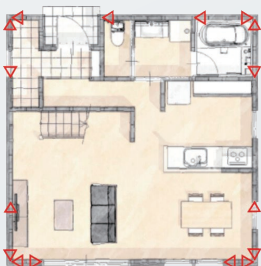
△：ダンパー設置位置
